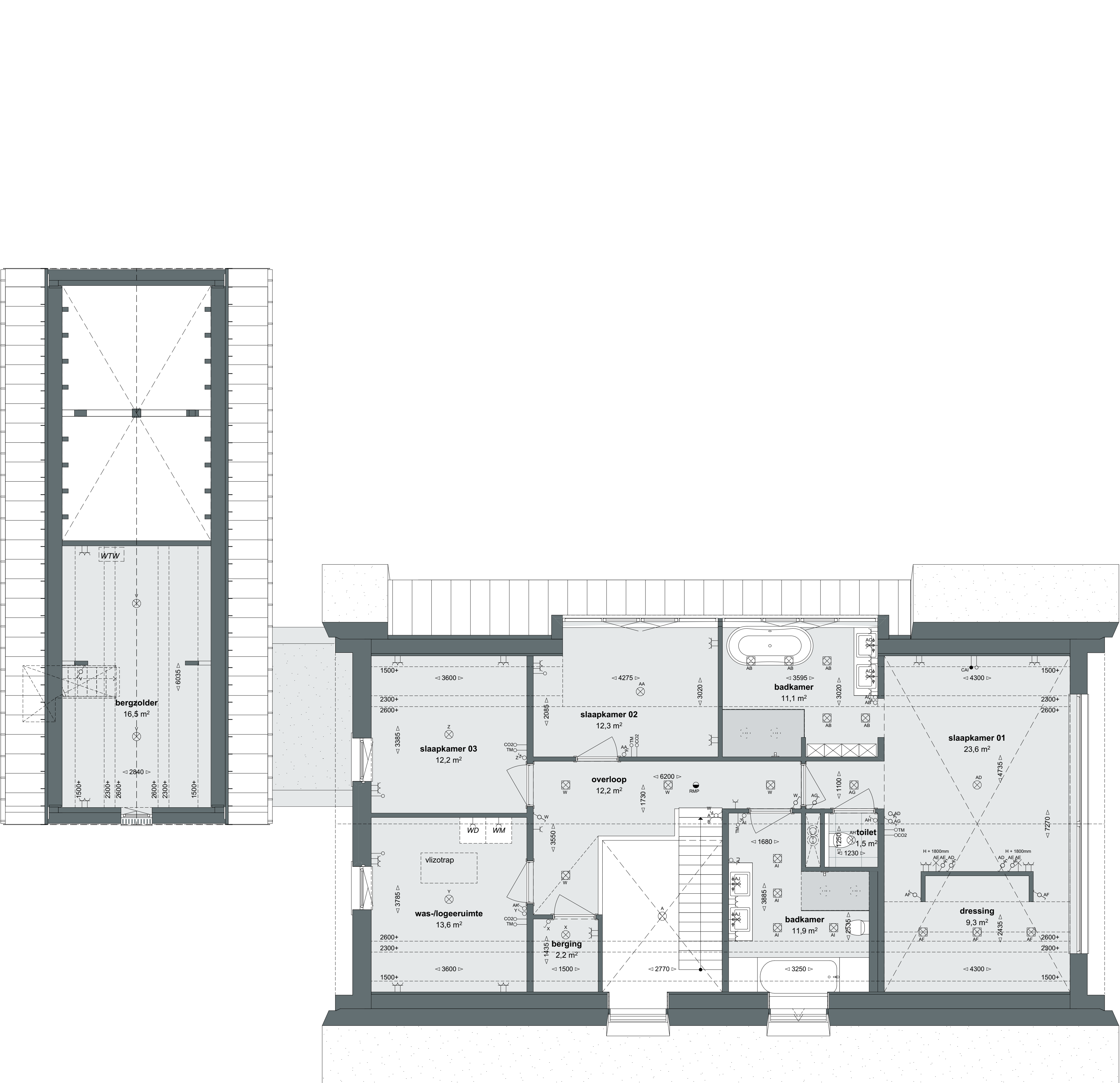
Eerste verdieping schaal 1:50
