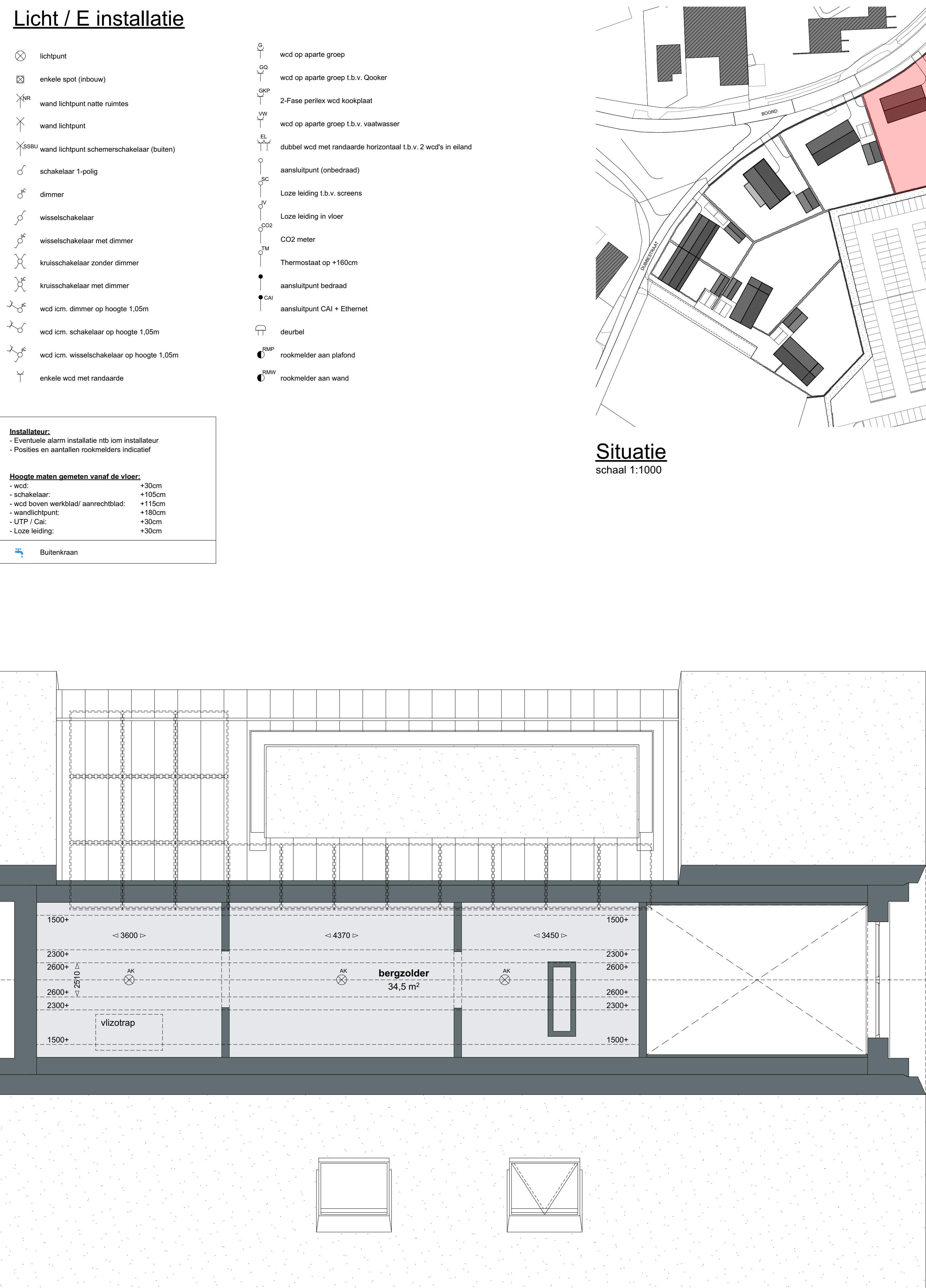
Tweede verdieping schaal 1:50
